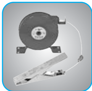
Pince renforcée en acier inoxydable Cen-Stat™ VESX90 et enrouleur rétractable de 15,2 m VESX90/R50
