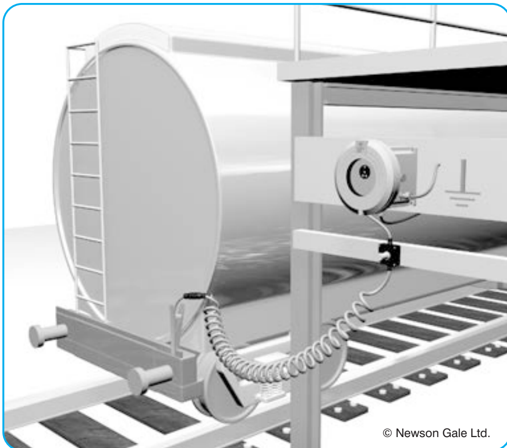
Earth-Rite PLUS avec câble spiralé de 10 m PLUSMEA1A3 - IECEX/ATEX PLUSMUA1A3 - Amérique du Nord
