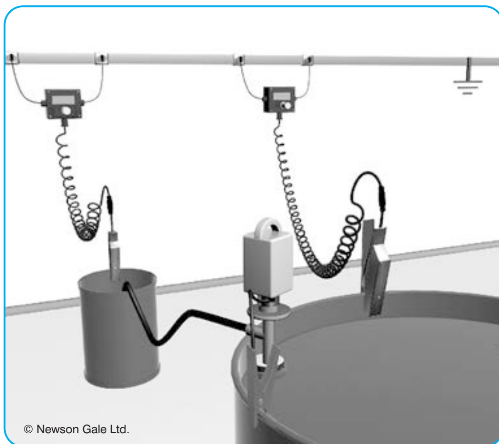
Pince de rechange Bond-Rite avec connecteur à détente rapide aligné VESC50
