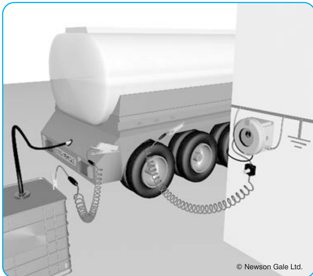
Bond-Rite EZ BREZ05/IPX90 - IECEX/ATEX BREZ05/IPX90 - Amérique du Nord
