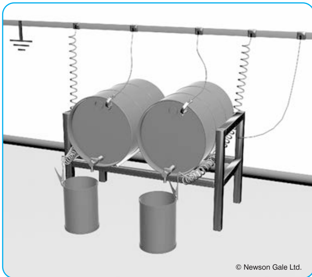
Pince en C et câble droit Cen-Stat™ VESC41/1GS01
