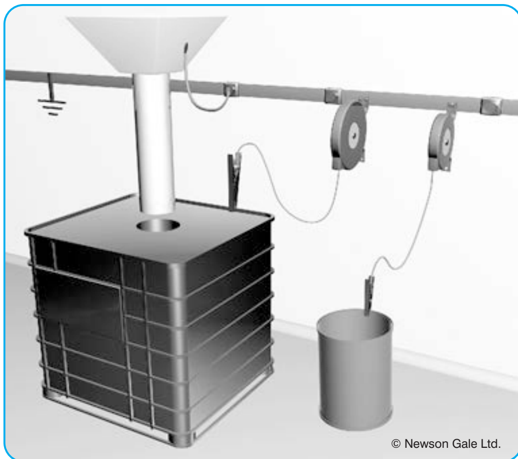
Pince renforcée en acier inoxydable Cen-Stat™ VESX90 et enrouleur rétractable de 15,2 m VESX90/R50
