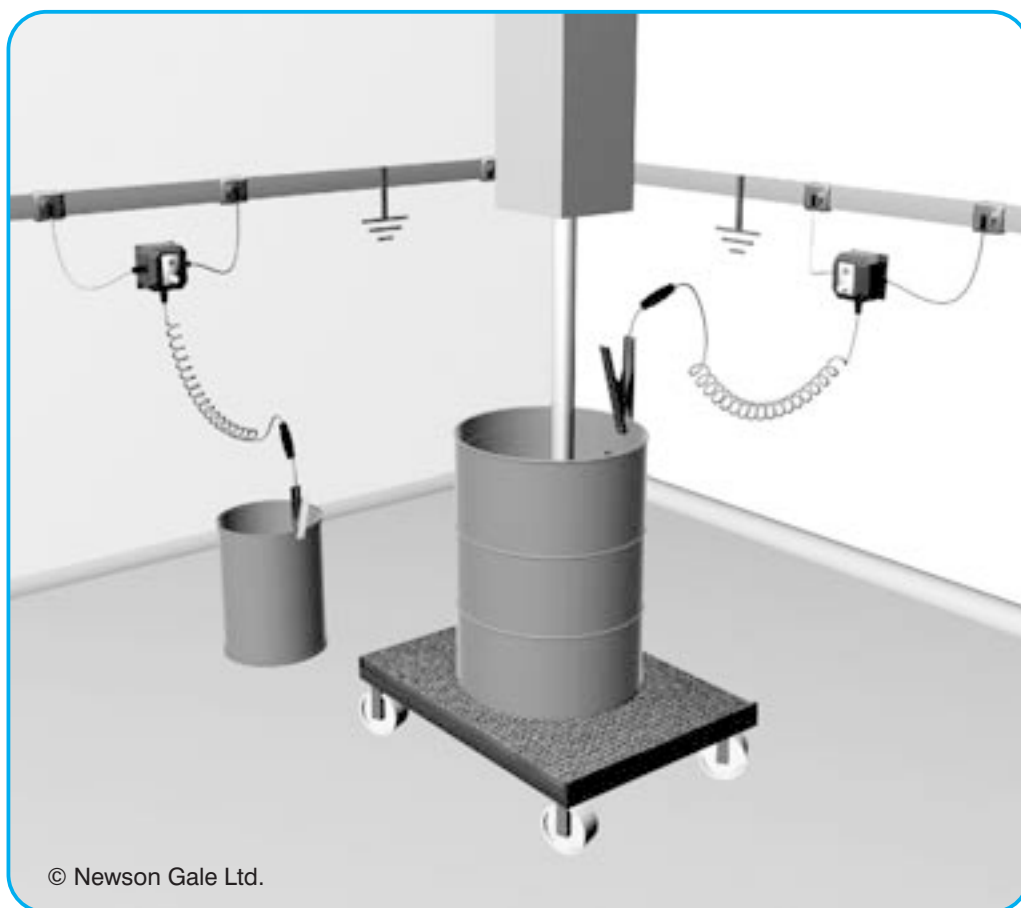
Bond-Rite REMOTE (boîtier en acier inoxydable) avec pince renforcée en acier inoxydable BRRMEB2A1- IECEX/ATEX BRRMUB2A1- Amérique du Nord
